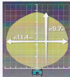
ML008Gの照射範囲 (照度70lx以上の範囲)
